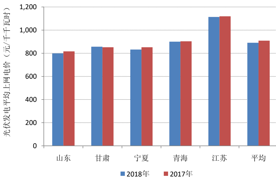
图 2-4 重点省份（地区）光伏发电平均上网电价
