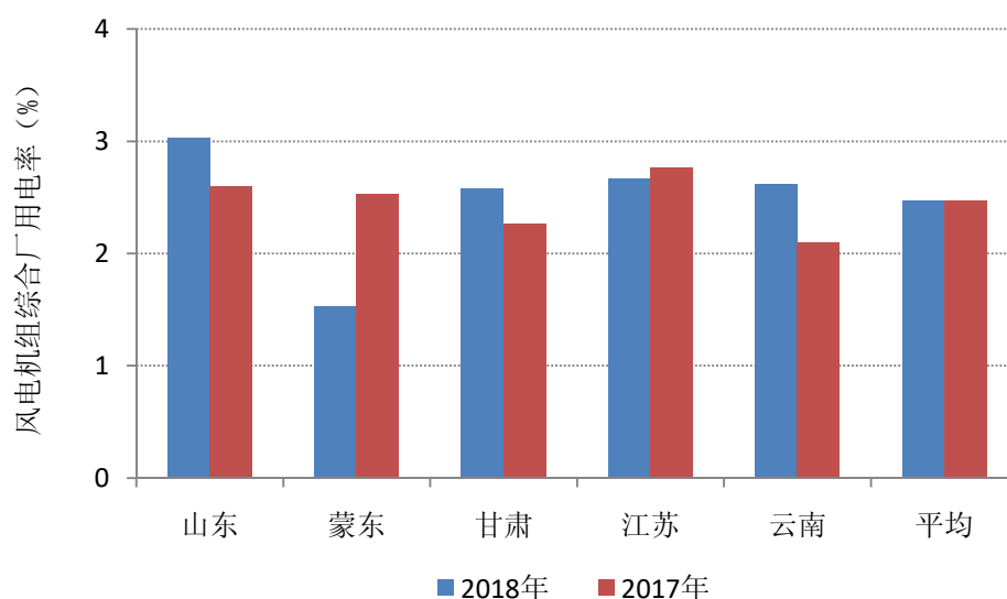
图 1-3 重点省份（地区）风电机组综合厂用电率
