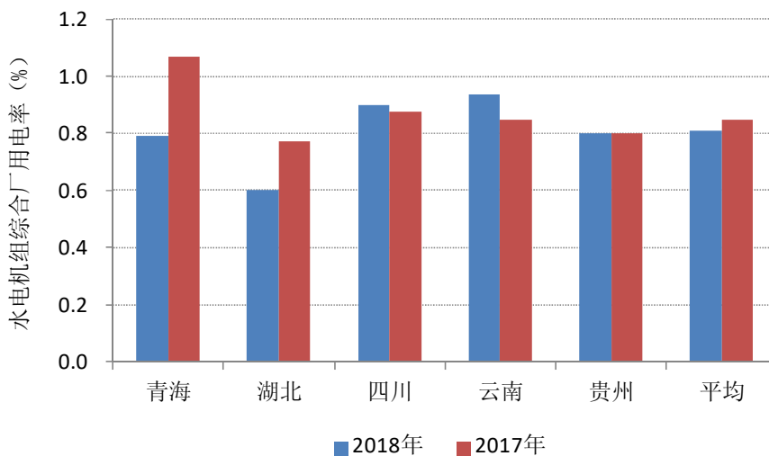
图 1-2 重点省份水电机组综合厂用电率
