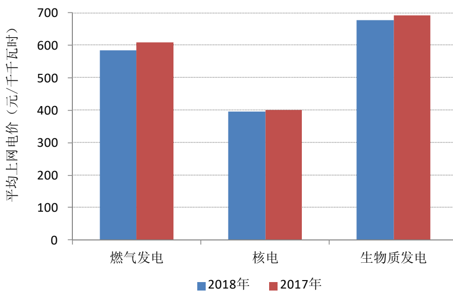
图 2-5 其他机组平均上网电价
