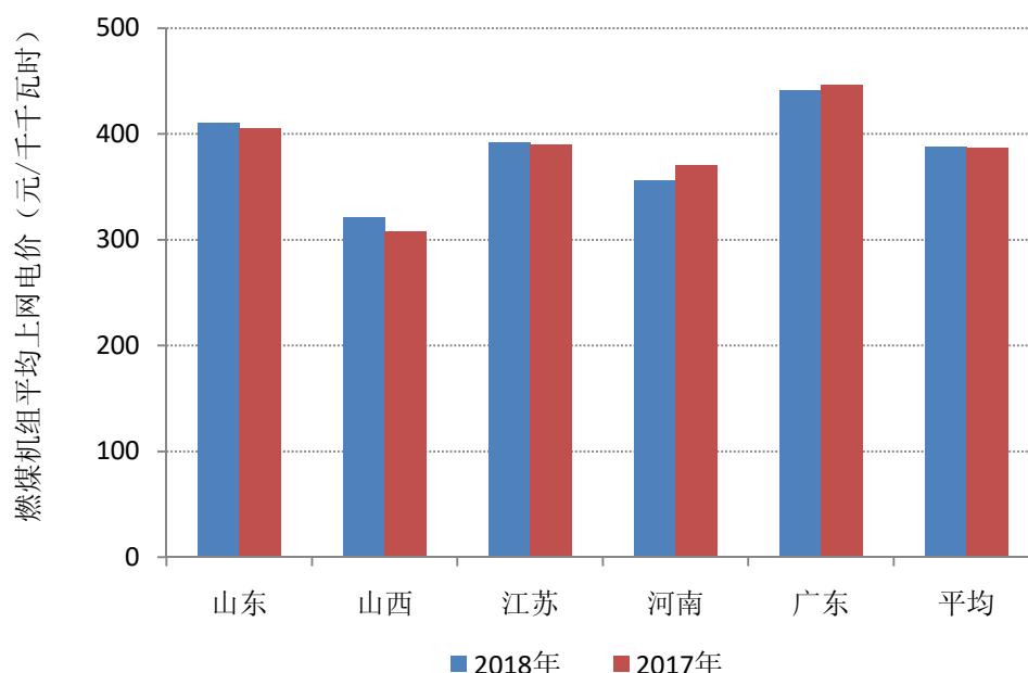
图 2-1 重点省份燃煤机组平均上网电价
