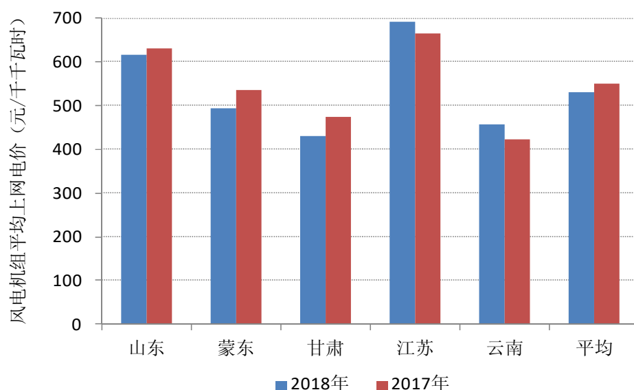
图 2-3 重点省份（地区）风电机组平均上网电价
