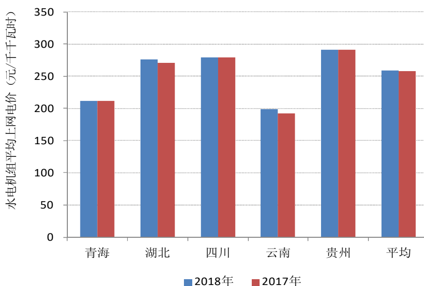
图 2-2 重点省份水电机组平均上网电价
