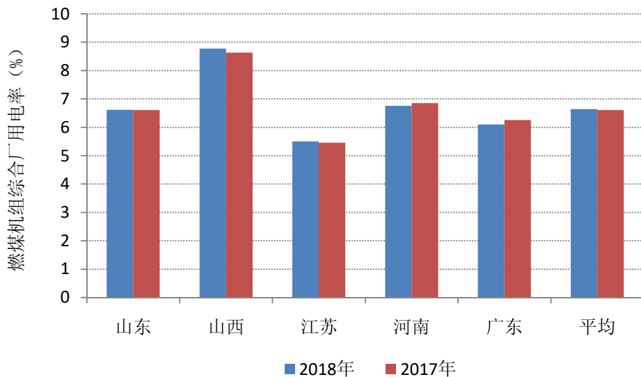
图 1-1 重点省份燃煤机组综合厂用电率
