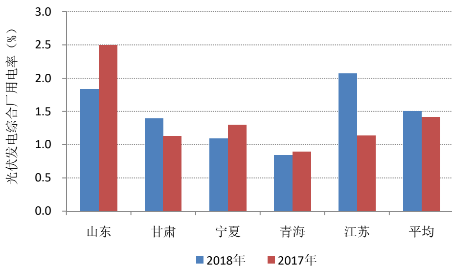
图 1-4 重点省份（地区）光伏发电综合厂用电率
